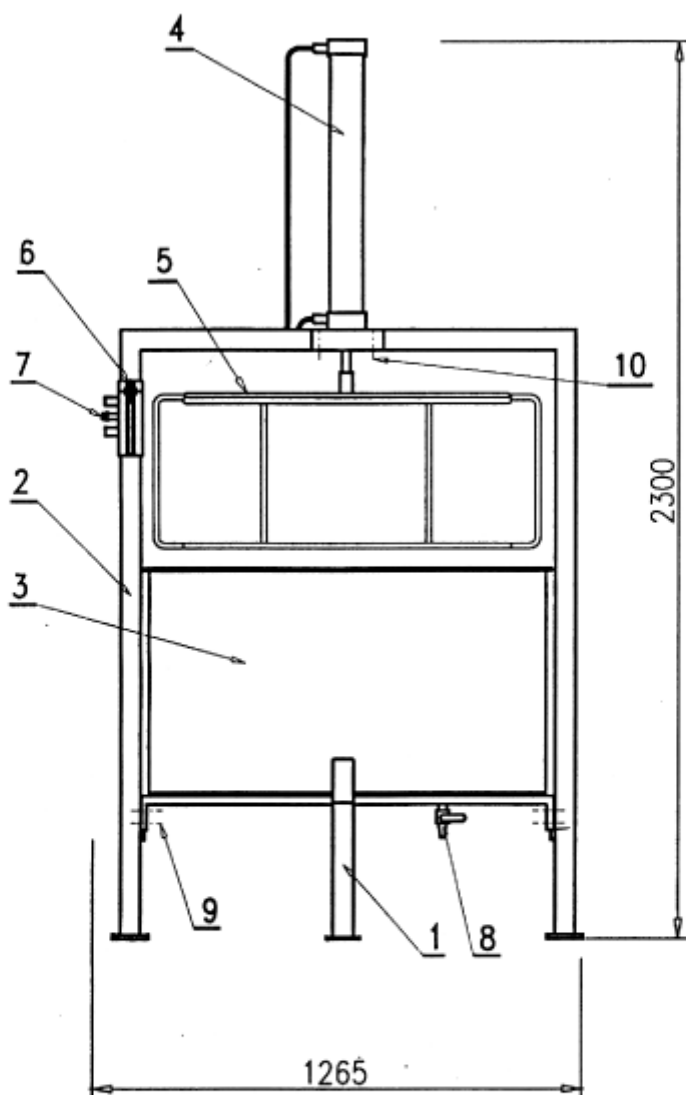
Rys.1. Wanna wulkanizatorska PNEUBAD-1
