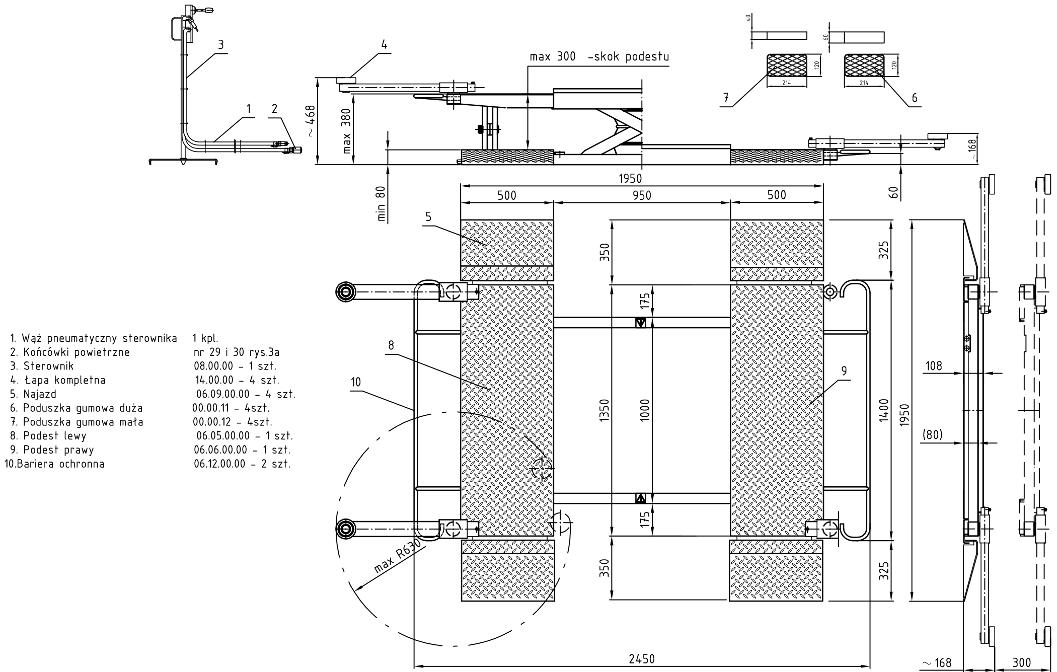
Rys. nr 1. Pneumatyczny podnośnik samochodowy typ PPS-5.
