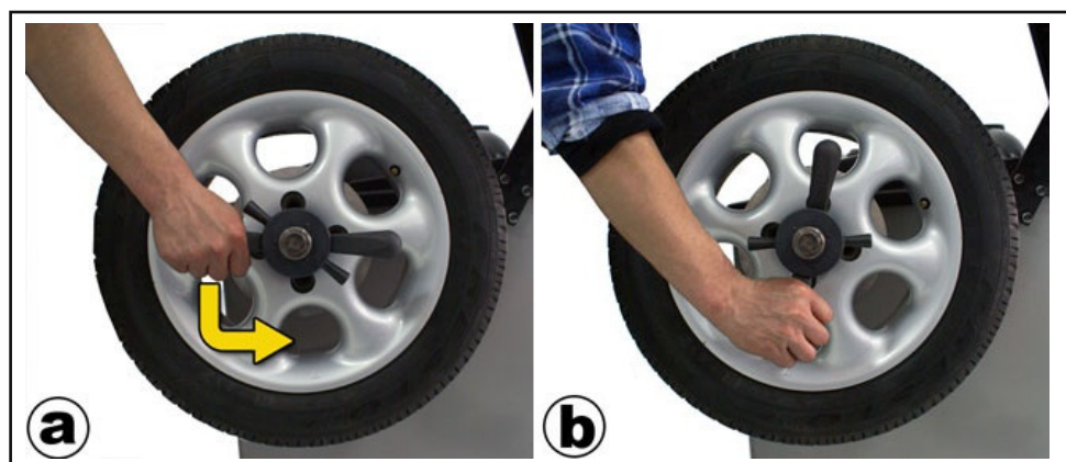
Rys. 5.8 Zdejmowanie koła z uchwyty wyważarki.
