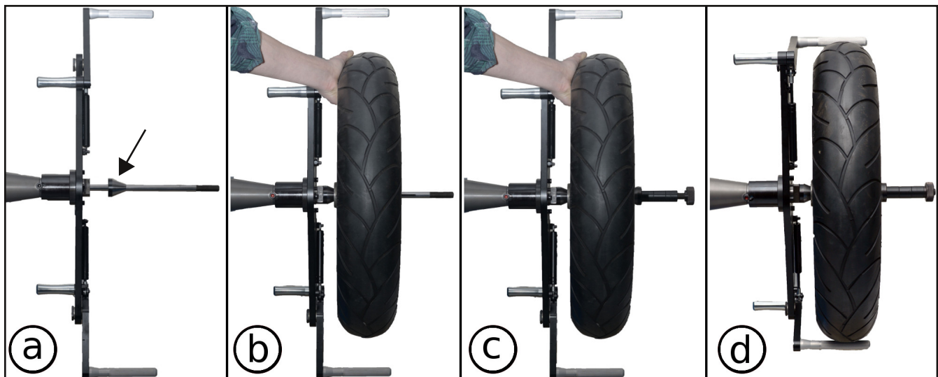
Rys. 5.13 Mocowanie koła motocyklowego w uchwycie.
