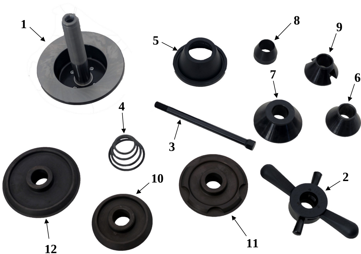
Rysunek 4: Elementy uchwyty: 1: nasada z flanszą 2: nakrętka dociskowa 3: śruba do mocowania nasady na wrzecionie 4: sprężyna 5: docisk nakrętki 6: stożek centrujący nr 1 7: stożek centrujący nr 2 8: stożek centrujący nr 3* 9: stożek centrujący nr 4* 10: stożek centrujący nr 5 (110mm-125mm)* 11: stożek centrujący nr 6 (125mm-145mm)*, 12: stożek centrujący nr 7 (145mm-165mm)* * - wyposażenie dodatkowe
